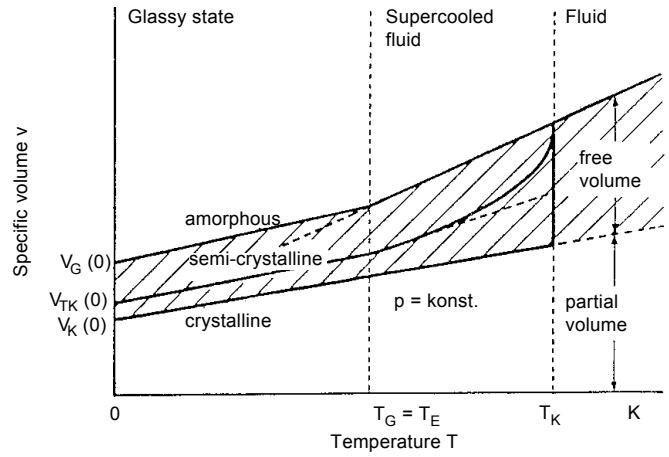
Fig. 5: Pressure-volume-temperature diagram (p-v- \vartheta -Diagram)
